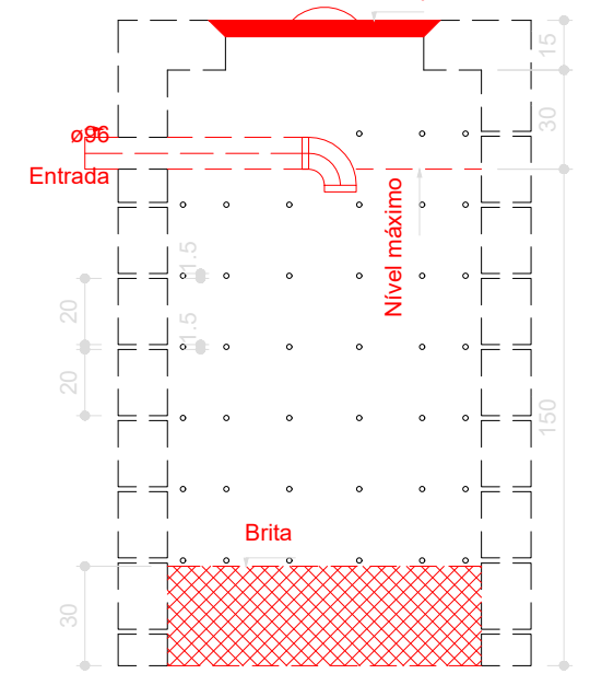
Sumidouro - Térreo Corte 1 - ESC. 1:25
