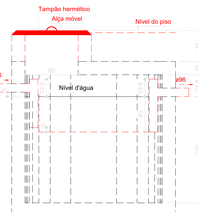
Tanque séptico - Térreo Corte 1 - ESC. 1:25
