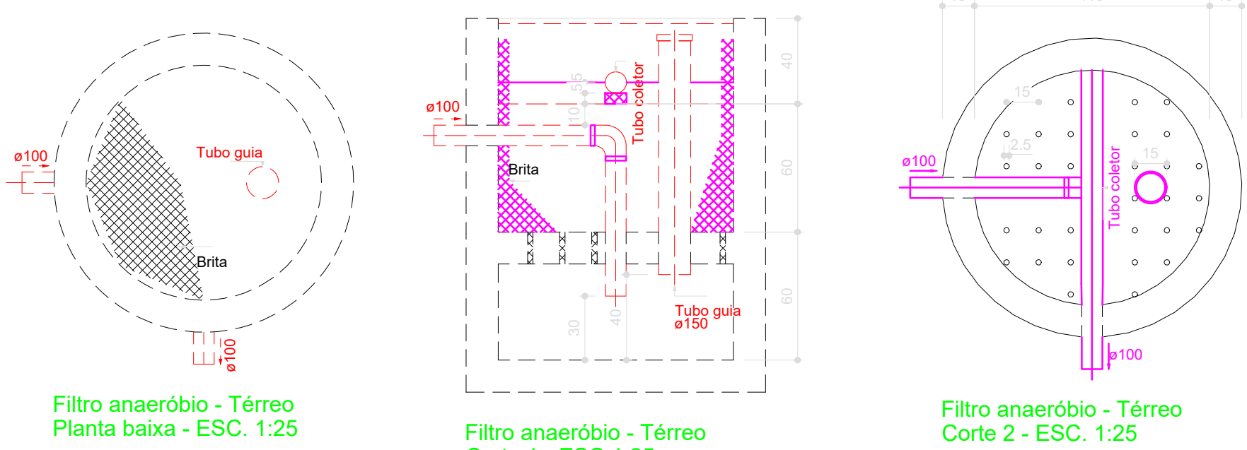
Filtro anaeróbio - Térreo Planta baixa - ESC. 1:25
