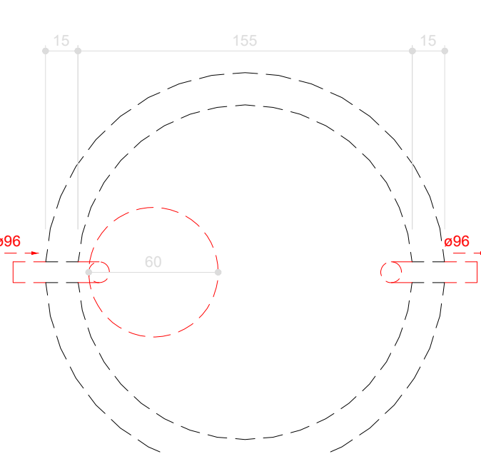
Tanque séptico - Térreo Planta baixa - ESC. 1:25
